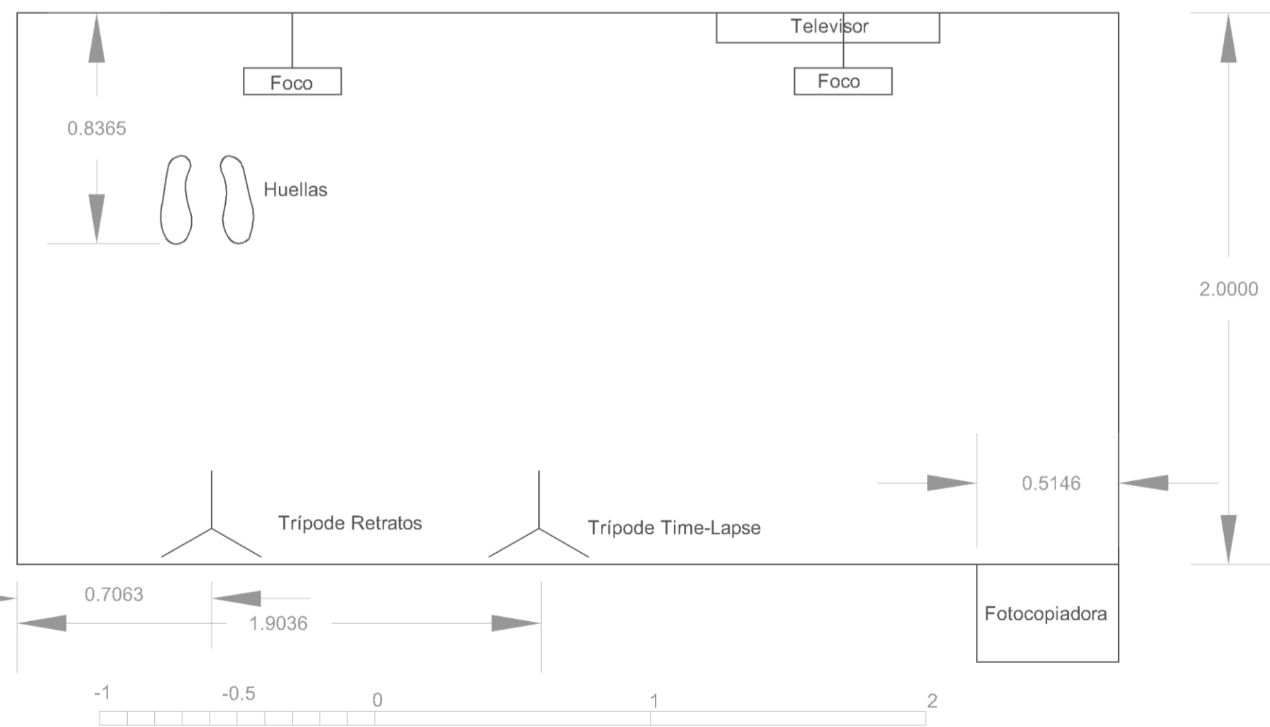
Alzado y planta de la exposición E 1:20
